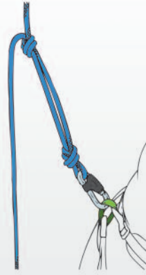
Anseilen in Seilweiche
