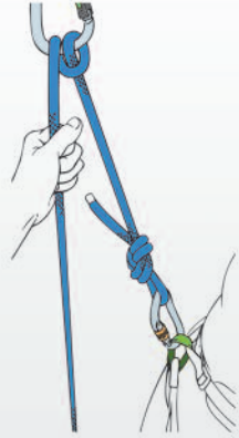
Verbindung Seil - Gurt beim Ablassen
